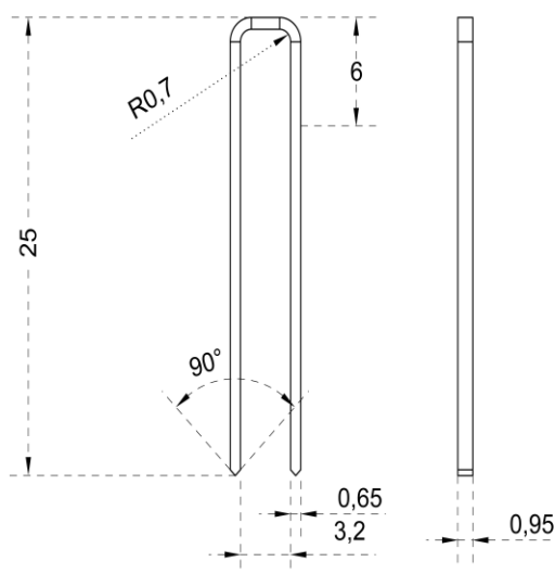
ΣΧΕΔΙΟ Ι: Σχήμα και Διαστάσεις σε mm των Συνδετήρων
